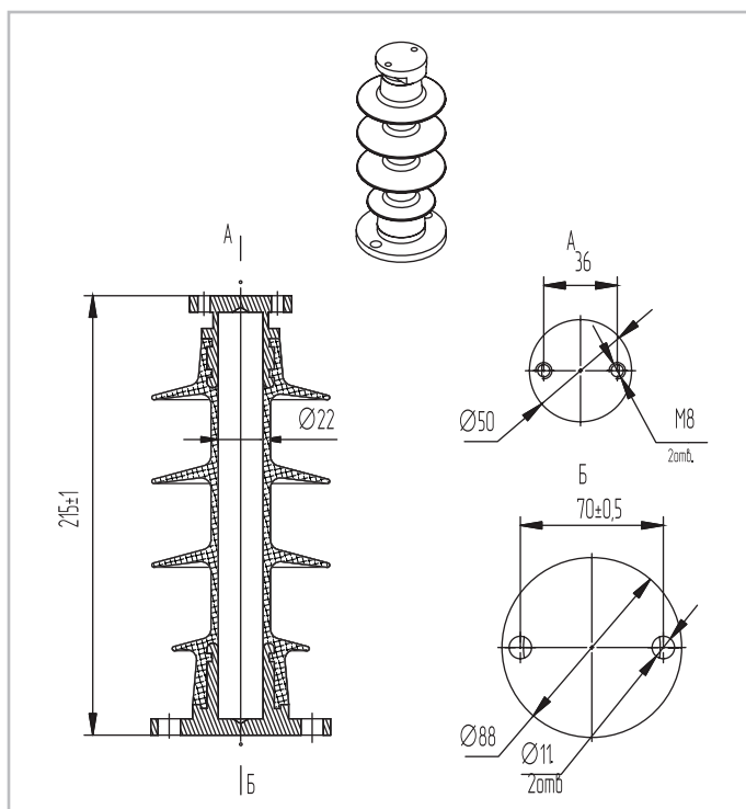
ОСК2-10-А-4 УХЛ1
