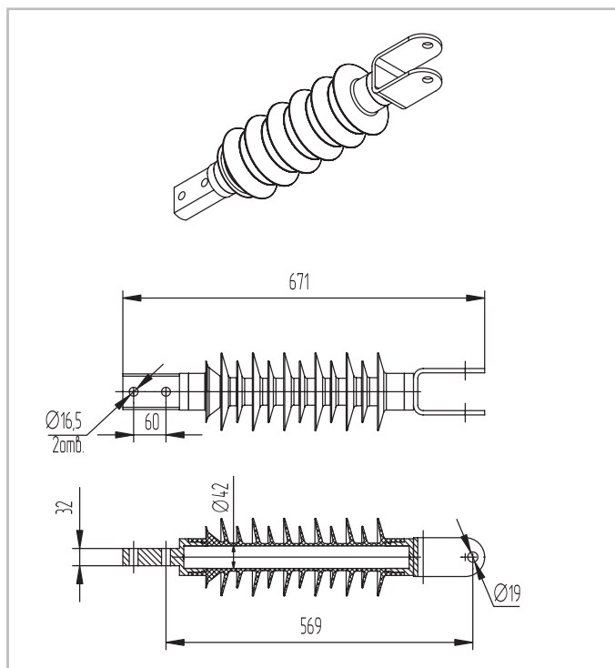
ОСК4-35-В-4УХЛ1
