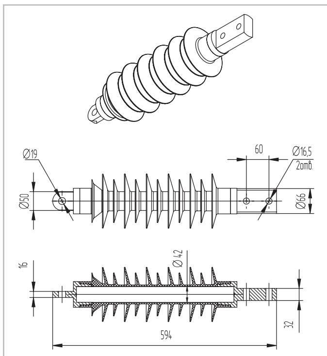
ОСК4-35-А-4УХЛ1
